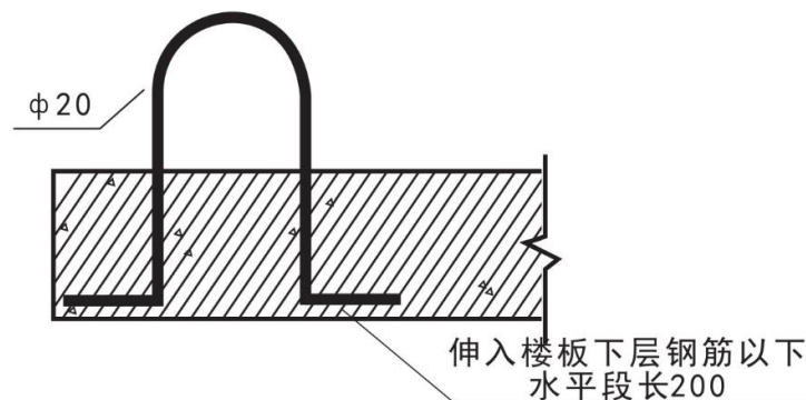
U形环埋设示意图
