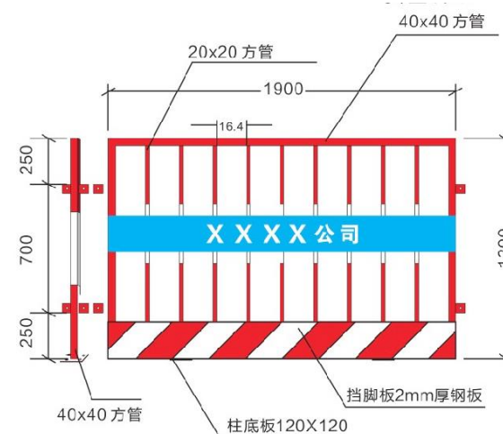
栏杆构造设计图（二）
