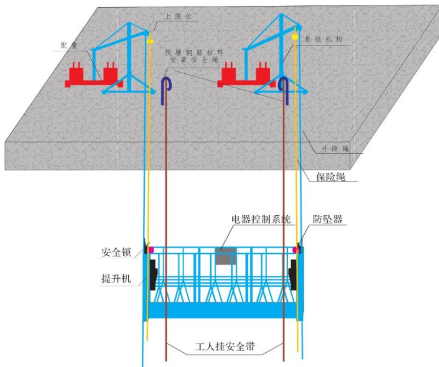
高处作业吊篮
