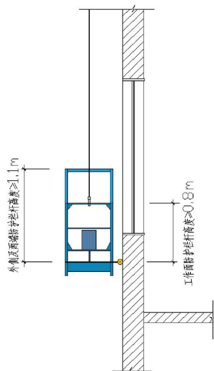
高处作业吊篮的护栏高度示意图
