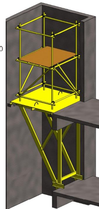
电梯井平台型式（四）
