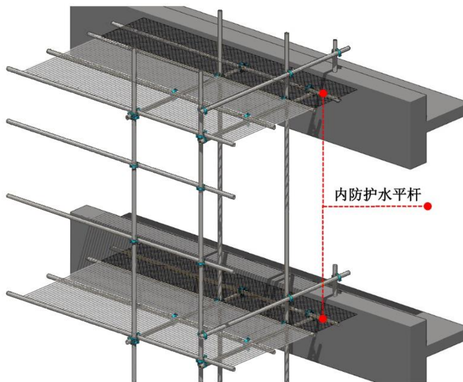
钢笆片防护
