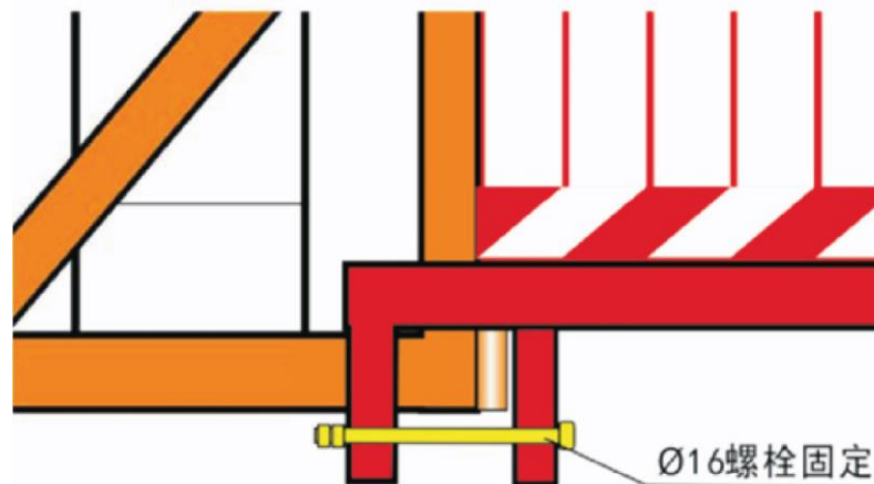
塔吊端采用挂钩形式
