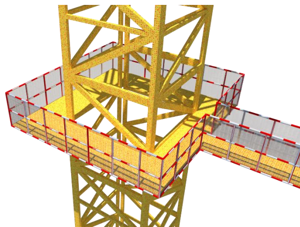
塔吊附墙操作平台示意图
