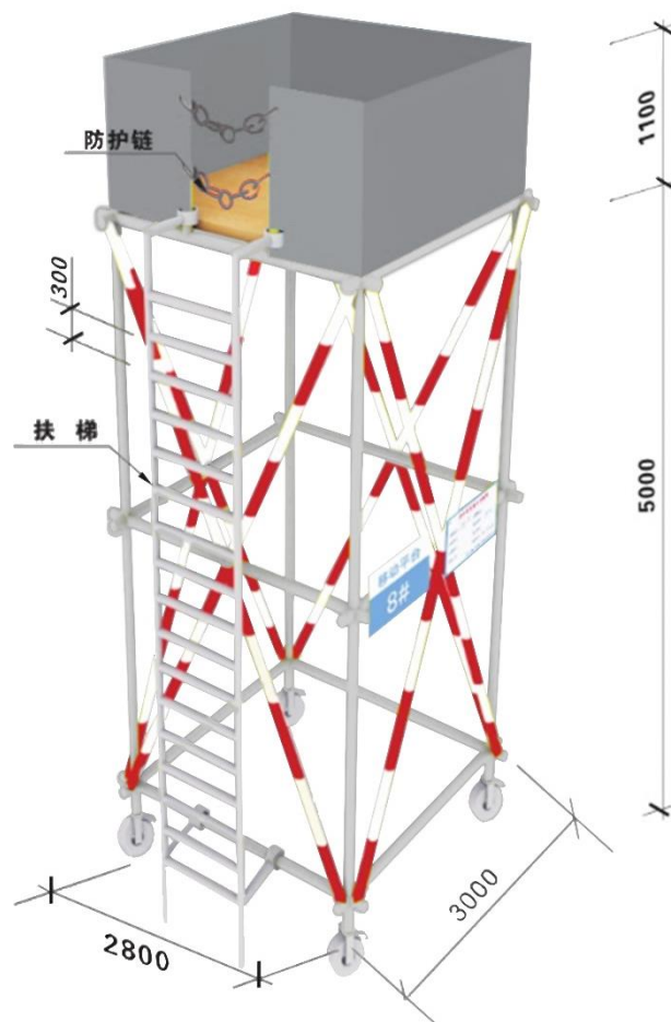
钢管脚手架移动式操作平台
