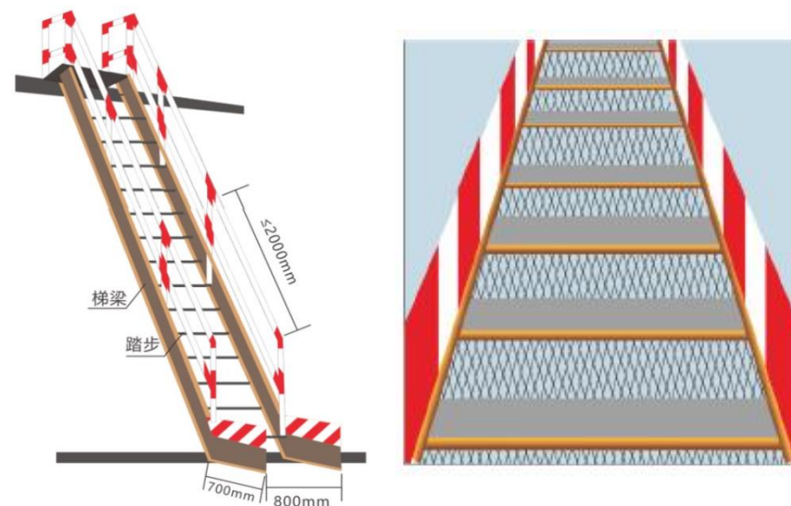
工具式爬梯
