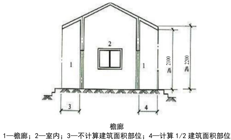
图 6.8 檐廊计算图示
